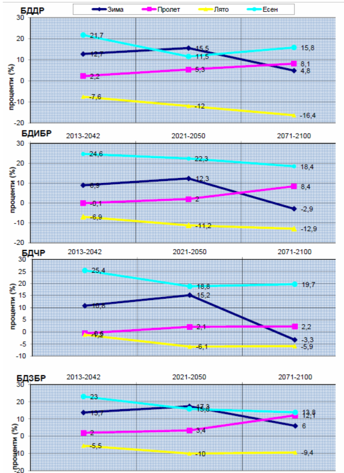
Фиг. 1.3. Средна разлика на валежните количества по сезони (%) спрямо периода 1976-2005 г. по сценария RCP 4.5
